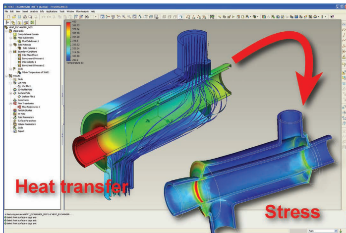
EFD2MECHANICA brengt de EFD thermische data over naar Pro/ENGINEER Mechanica voor de structurele analyse
